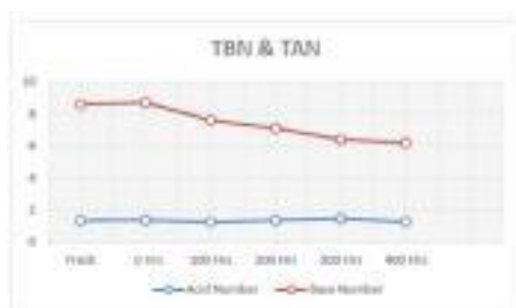
Figure 3 Volvo D12
